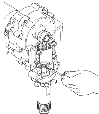
Fig. 2. Empuje hacia arriba el anillo de retención (26).
