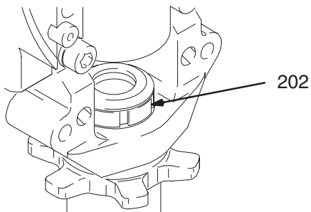
Fig. 7. Saque la tuerca prensaestopas (202).
