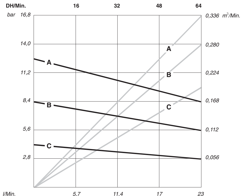
FÖRDERLEISTUNG (TESTFLÜSSIGKEIT: MOTORÖL NR. 10)
