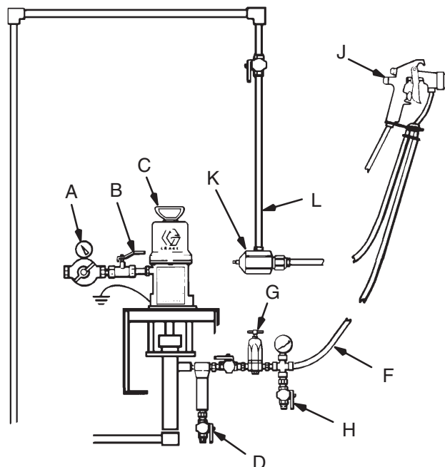
Estação de pulverização de circulação única
