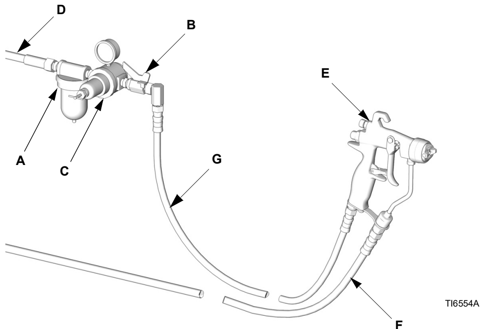
FIG. 1 : Installation type (illustration modèle G15)
