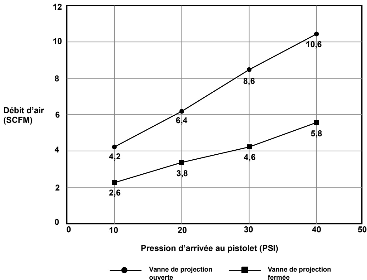
Débit d'air, Chapeau d'air standard série AA
