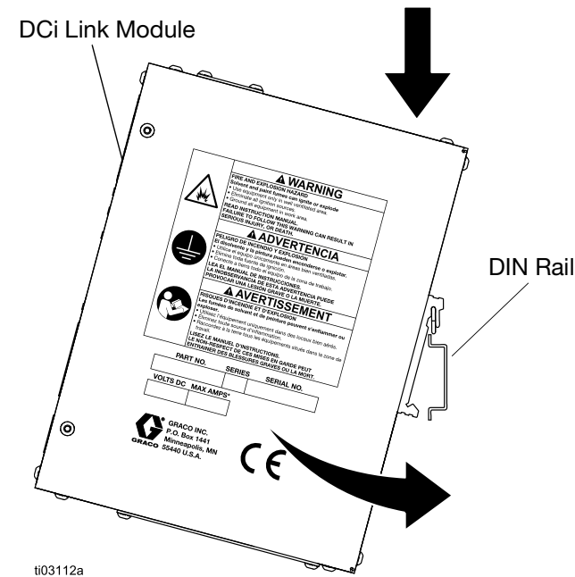
ti03112a Fig. 3: Mount Module on DIN Rail
