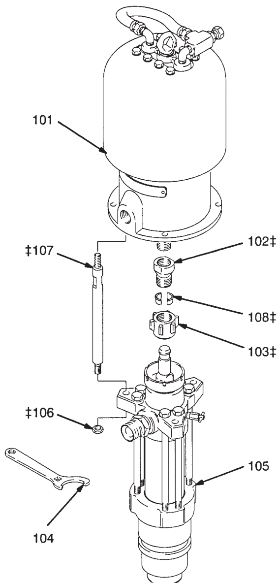
Modell 222-905 Serie A 24:1 King Pumpe mit schallgedämpftem Luftmotor
