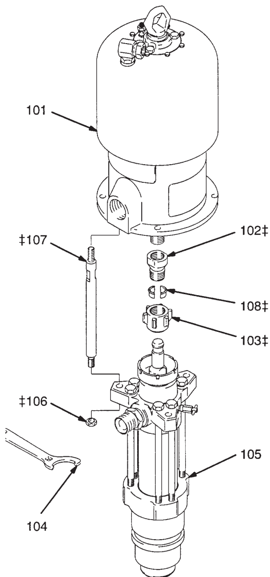
Modell 222-836, Serie A 24:1 King Pumpe mit Standard Luftmotor
