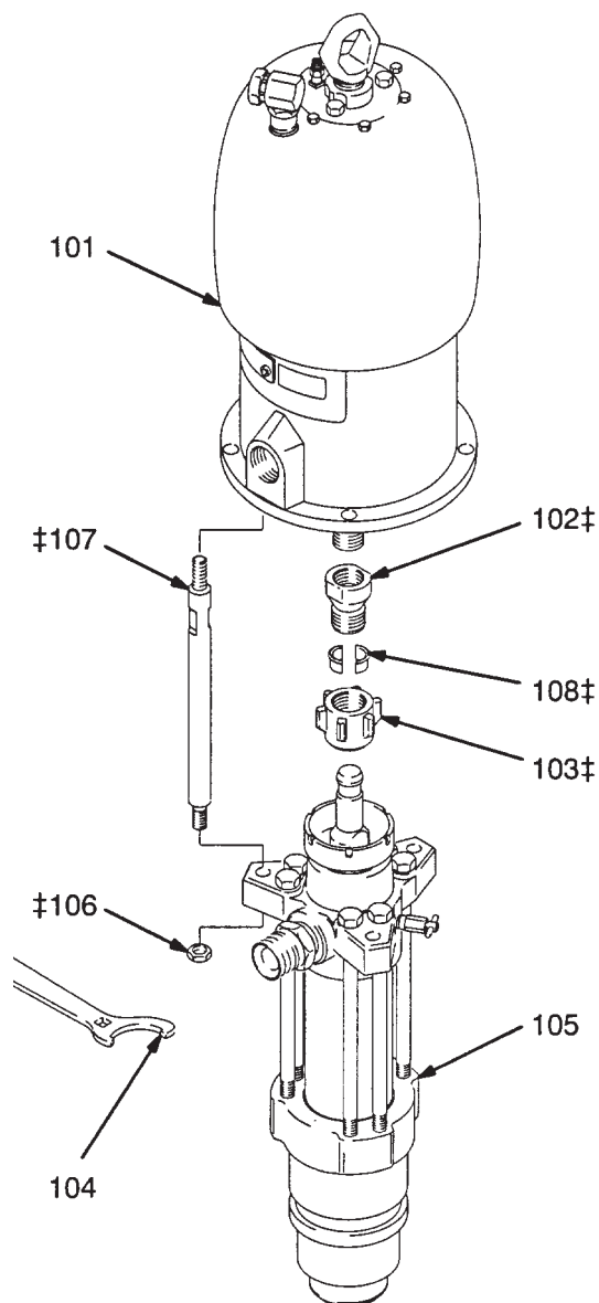
Modell 222-904, Serie A 12:1 Bulldog Pumpe mit Standard Luftmotor
