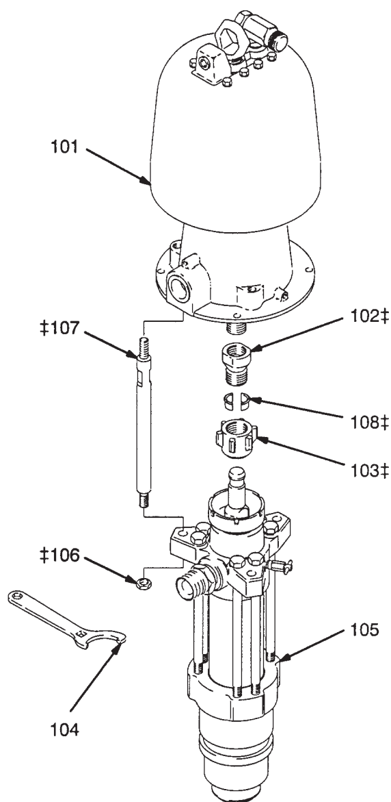
Modell 222-903, Serie A 12:1 Bulldog Pumpe mit schallgedämpftem Luftmotor
