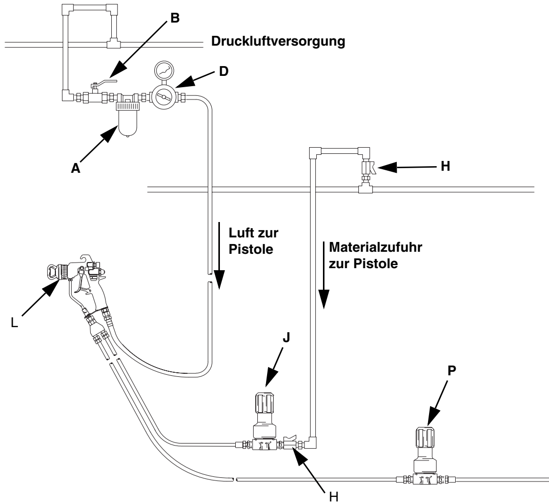
Fig. 6. Mechanischer Hochdruck-Regler und Gegendruckregler für Nicht-Zirkulationssystem Zeichenerklärung
