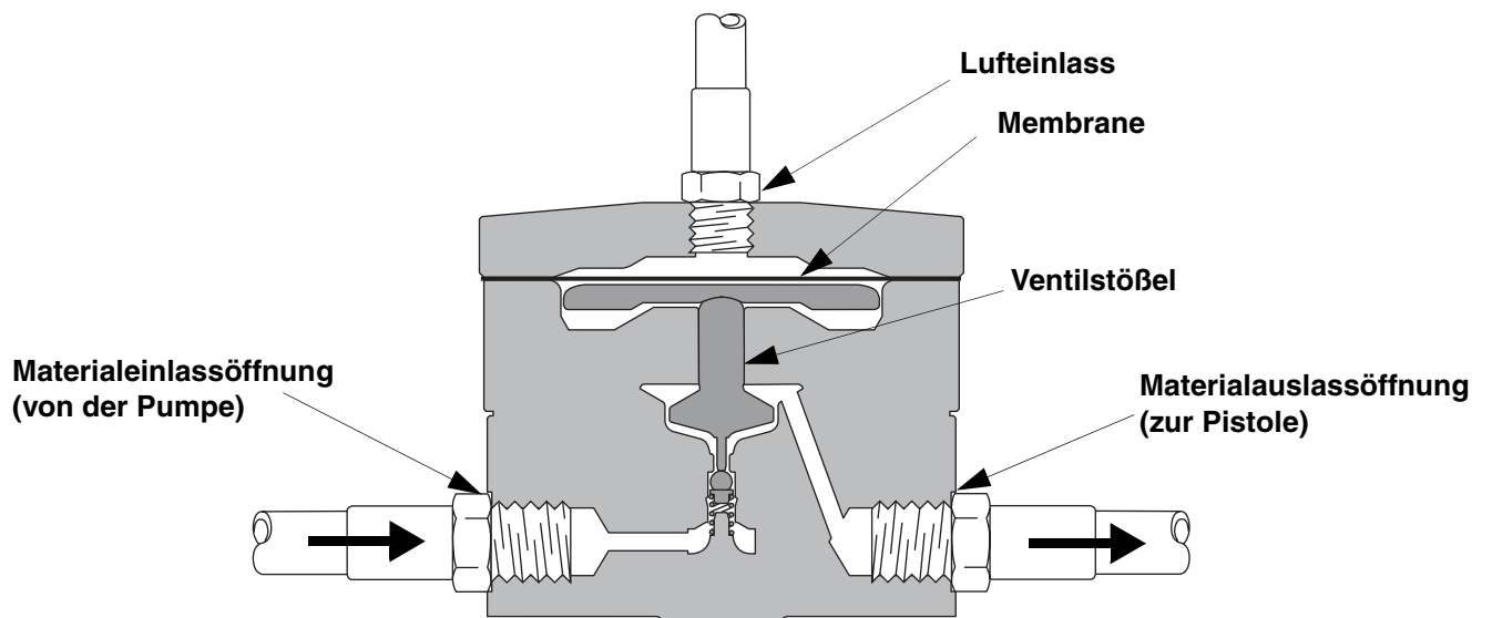
Fig. 2. Schnittansicht eines mechanischen Druckreglers
