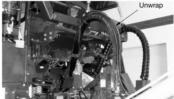
FIG. 104: HM300-5
