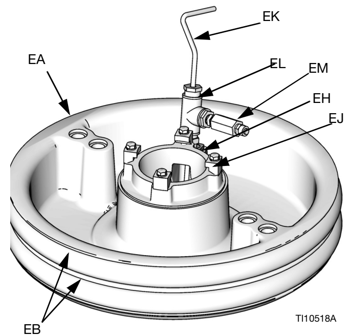
FIG. 3. Platen
